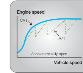
فتيس أوتوماتيك CVT CVT AT TRANSMISSION
